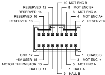
Incremental Encoder
